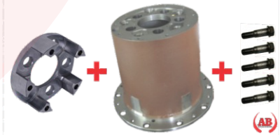
AB-M 07 VAZIA AB-M 18 - Cubo Planetário de Redução - "Cartola" * (Montada)
